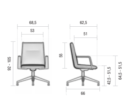
Giratoria Giratória / Giratoire / Swivel / Drehstuhl.
