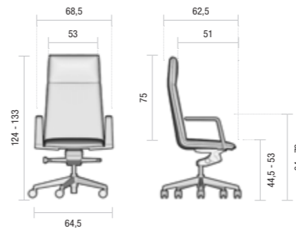
Silla de dirección Cadira de direcció / Siège direction / Executive chair / Chefessel Stuhl.
